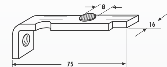
30306 A Ø = 7,5 mm
