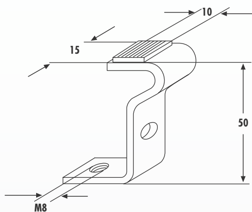
30619 Pasticca spessore 3 mm Auflegestärke 3 mm Pastille thickness 3 mm Pastille épaisseur 3 mm
