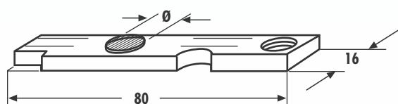
30303 A Ø = 7,5 mm
