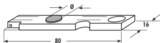
30302 A Ø = 7,5 mm
