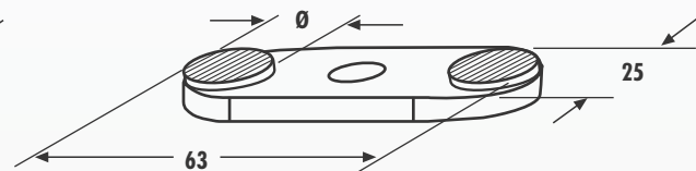
30312 A Ø = 7,5 mm
