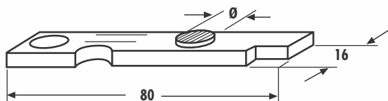
30301 A Ø = 7,5 mm
