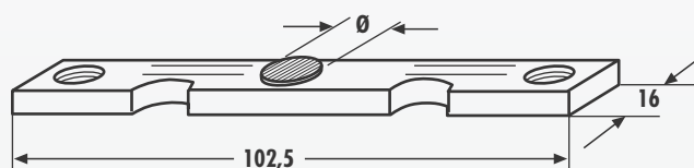
30307 A Ø = 7,5 mm
