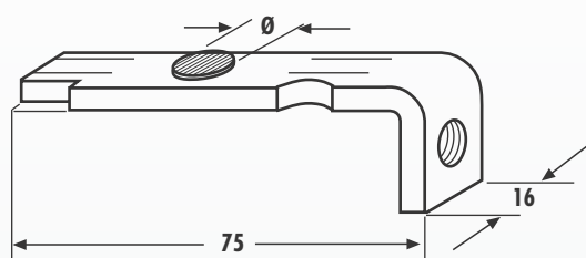
30305 A Ø = 7,5 mm
