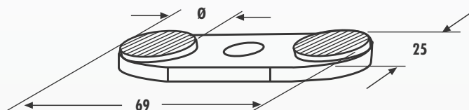
30323 A Ø = 10 mm
