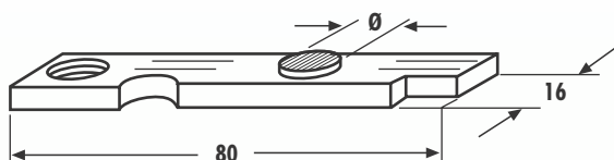
30304 A Ø = 7,5 mm
