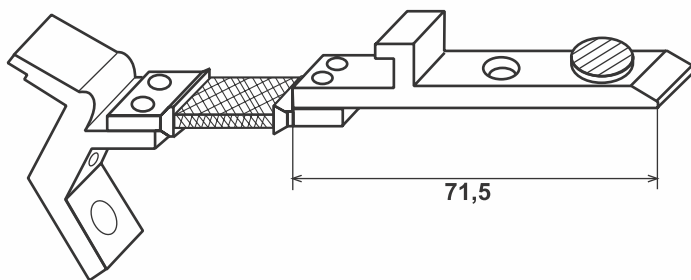
30101 con molla / mit Feder / with spring / avec ressort
