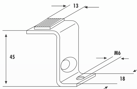
30620 Pasticca spessore 1 mm Auflegestärke 1 mm Pastille thickness 1 mm Pastille épaisseur 1 mm
